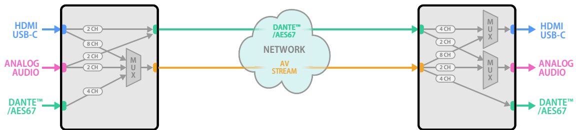
DuetE-5 • Encoder
