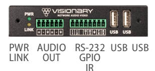
DuetD-2 • Decoder
