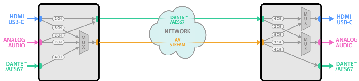
DuetE-2 • Encoder
